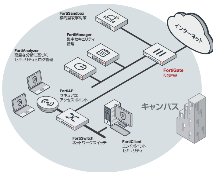
FortiGate 800D のキャンパスへの導入例 (NGFW)
