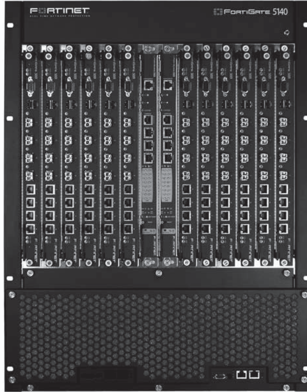
FortiGate-5140シャーシ(前面)
