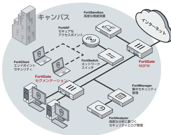
FortiGate 3900E シリーズの大規模なキャンパスへの導入例 (NGFW、インテント ベースト セグメンテーション)
