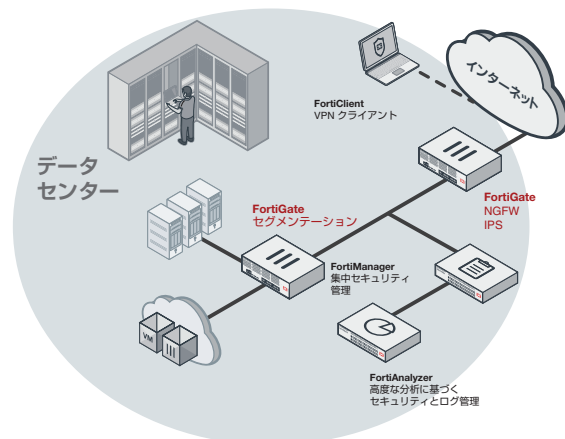
FortiGate 3700D のデータセンターへの導入例 (IPS / NGFW、インテント ベースト セグメンテーション)
