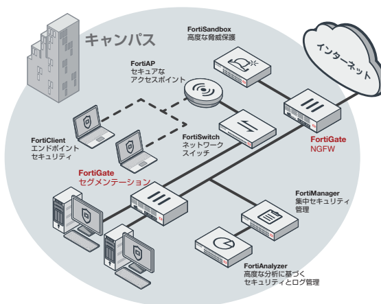
FortiGate 3700D の大規模なキャンパスへの導入例 (NGFW、インテント ベースト セグメンテーション)
