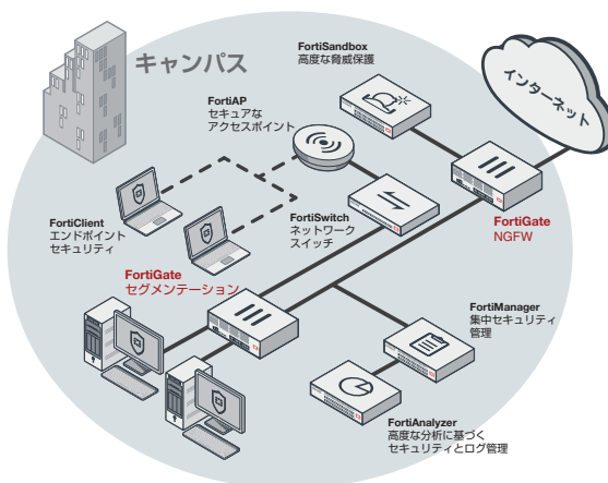
FortiGate 3600E の大規模なキャンパスへの導入例 (NGFW、インテント ベースト セグメンテーション)
