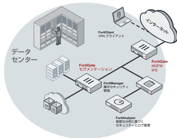
FortiGate 2500E のデータセンターへの導入例 (IPS / NGFW、インテント ベースト セグメンテーション)
